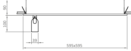
Tavan Tipi-Montaj Ölçüsü
