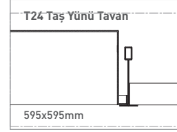
Tavan Tipi-Montaj Ölçüsü
